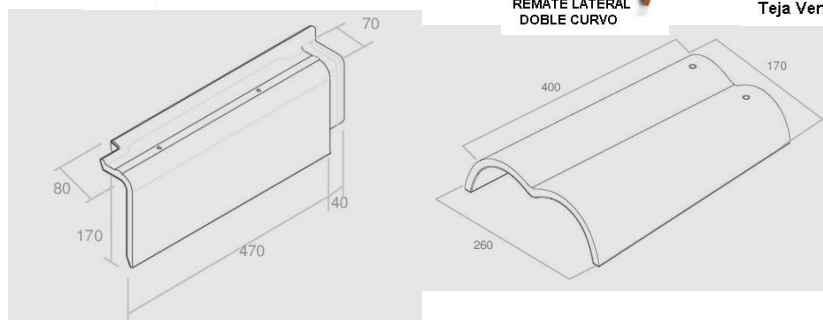
Teja Ventiladora
